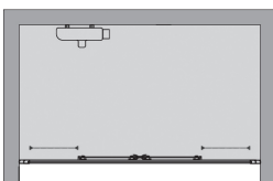
Liukuseinä alaliukukiskolla
